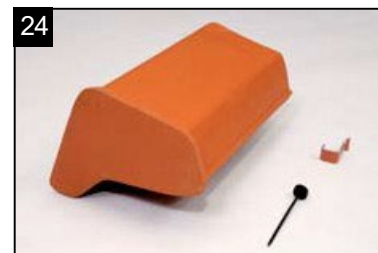
24 SET univerzální pultový hřebenáč zakočovací, levý s jednou přichytkou hřebenáče HO + N a s jedním vrutem Pro napojení pultové hrany na štítovou.
